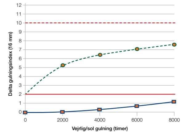
Gulningsindex. Data fra ATLAS Ci5000 (ISO 11341 / ASTM G155) om vejrlig.
