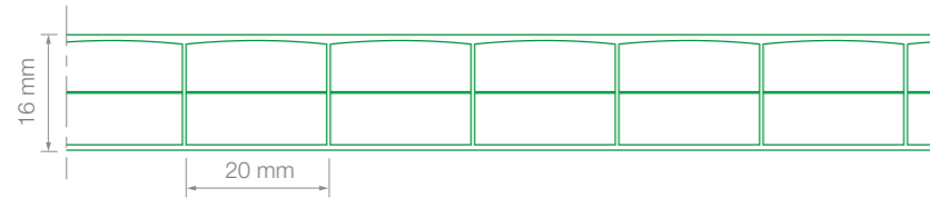
16 mm/3 lag
