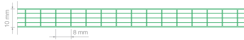
10 mm/5 lag
